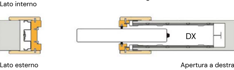
Apertura scorrevole a scomparsa (pratica) Sliding door – Coulissante modèle
